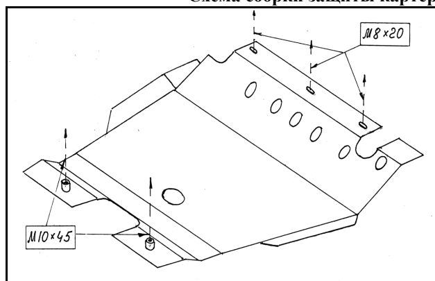
Схема сборки защиты картера и КПП.
