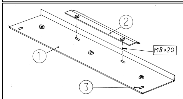
Установка защиты
